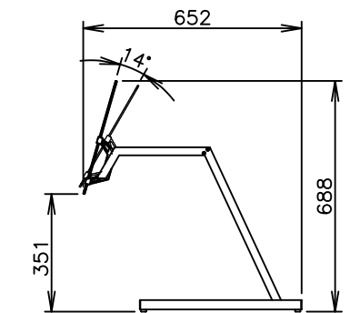
フロントガード：角度変更(14°) (尺度：1：2)
