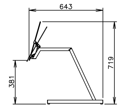
フロントガード：アップ+角度変更(14°) (尺度：1：2)
