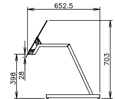
フロントガード：アップ (尺度：1：2)
