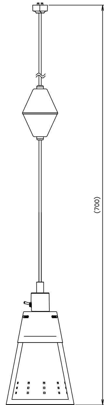
コード長 Ver.1 (縮めた状態)
