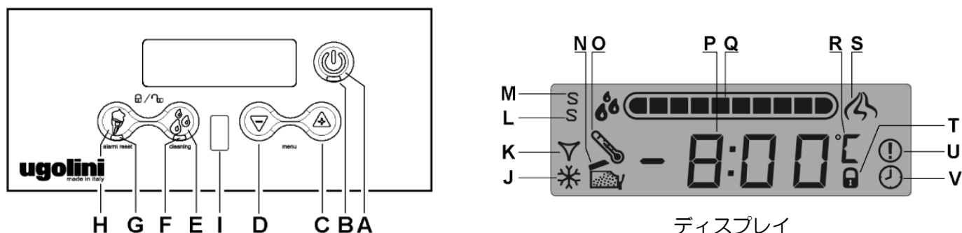
図1 操作キーパッド
